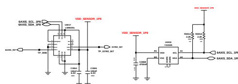
6 AXIS(ACC+GRYO)
